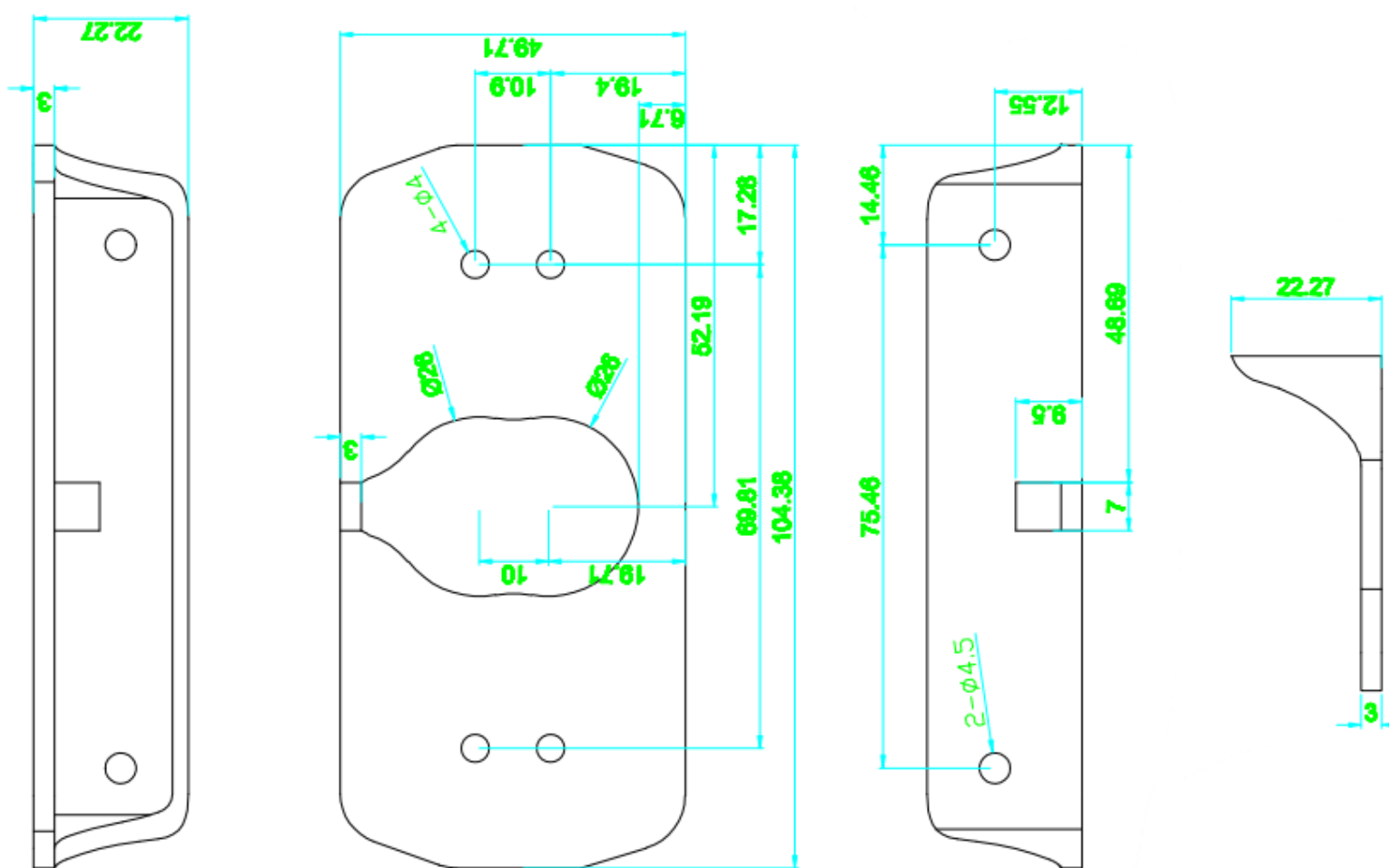
Plan patte droite-equerre pour feu de position rectangulaire
